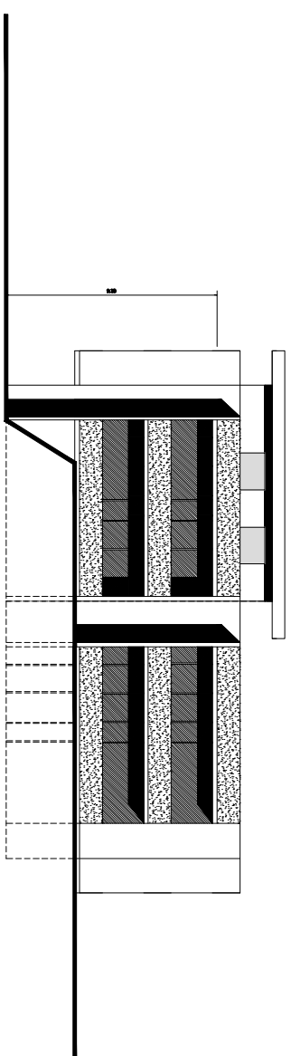
prospetto laterale C
